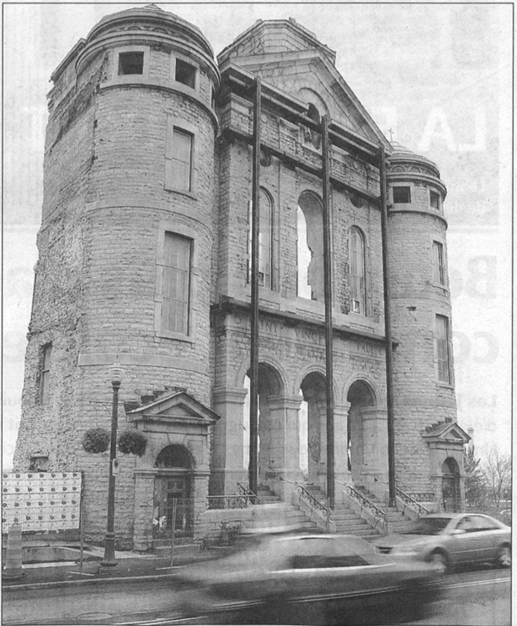
Un ingénieur a conclu qu'il était possible de consolider la façade avec des poutres de soutènement en acier durant la construction. — PHOTO LE SOLEIL, ERICK LABBÉ
